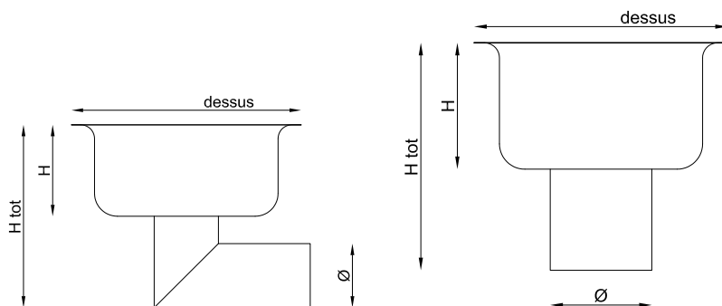
EKO, siphon de sol en inox AISI 304, exécution mate avec sortie verticale
