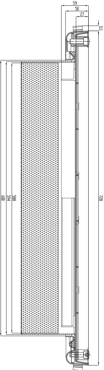
A-A
