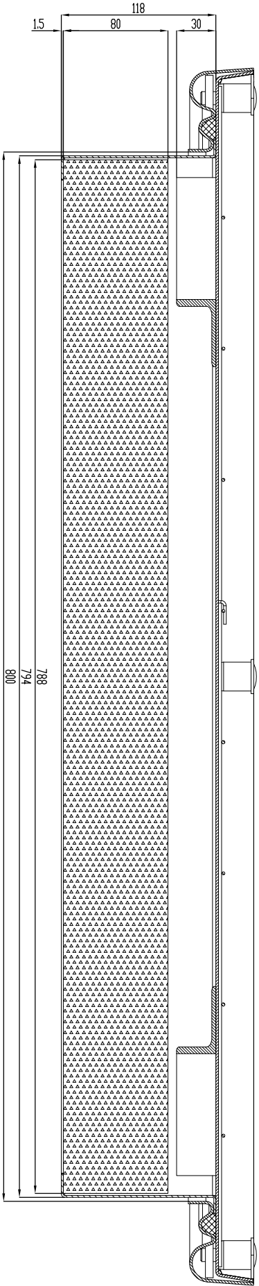
B-B
