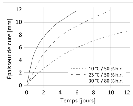
Diagramme 1: vitesse de polymérisation du Sikaflex®-268
