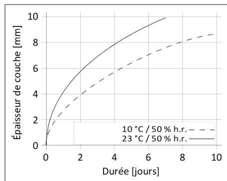
Diagramme 1: Vitesse de durcissement de SikaTack® PRO
