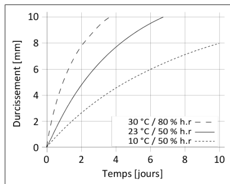
Diagramme 1 : Vitesse de polymérisation du Sikaflex®-263
