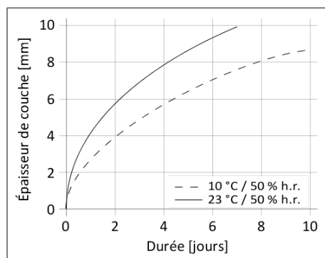
Diagramme 1: Vitesse de durcissement de SikaTack® MOVE Transportation
