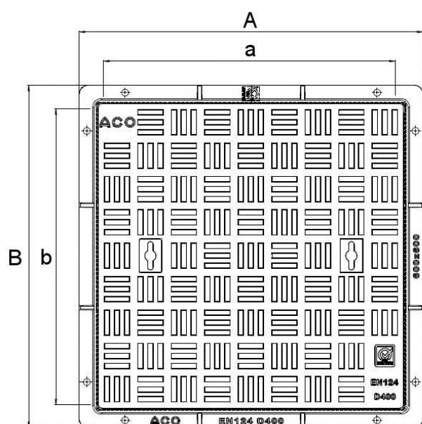
Rectop couvercle hydraulique 600x600 mm
