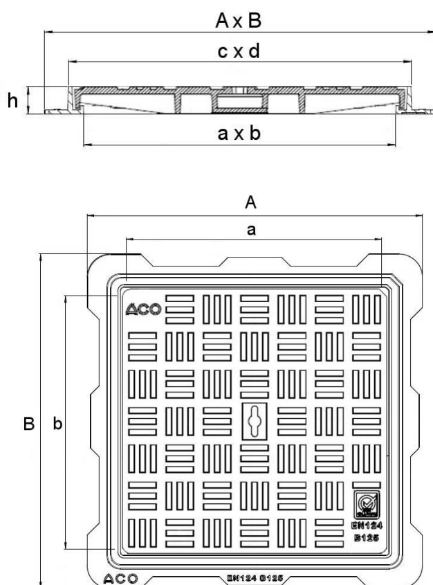
Rectop couvercle hydraulique 500x500 mm
